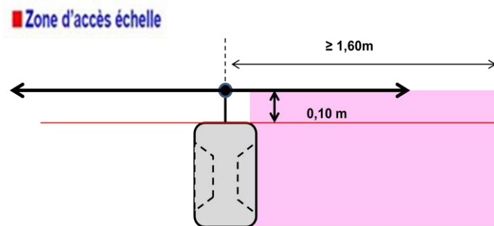
Figure 9 – Zone d'accès échelle sur Réseau HTA
